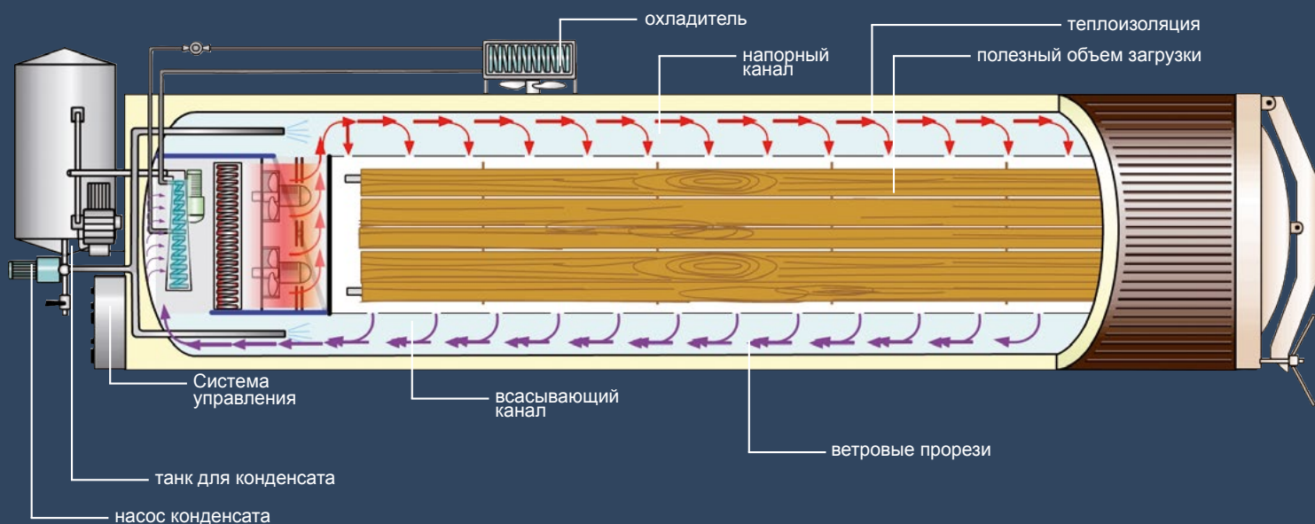
Сушильная камера в момент циркуляции, графическое изображение в поперечном сечении, вид сверху.
